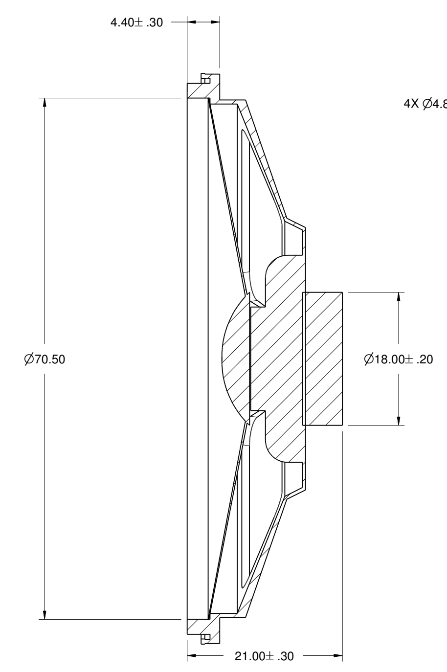
Section A-A
